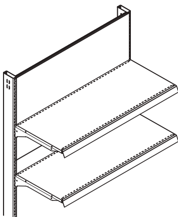
Fijado a la pared
